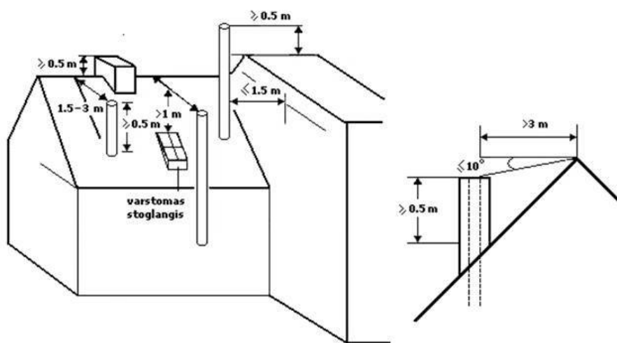
2 paveikslas. Dūmtraukių išdėstymo principas
